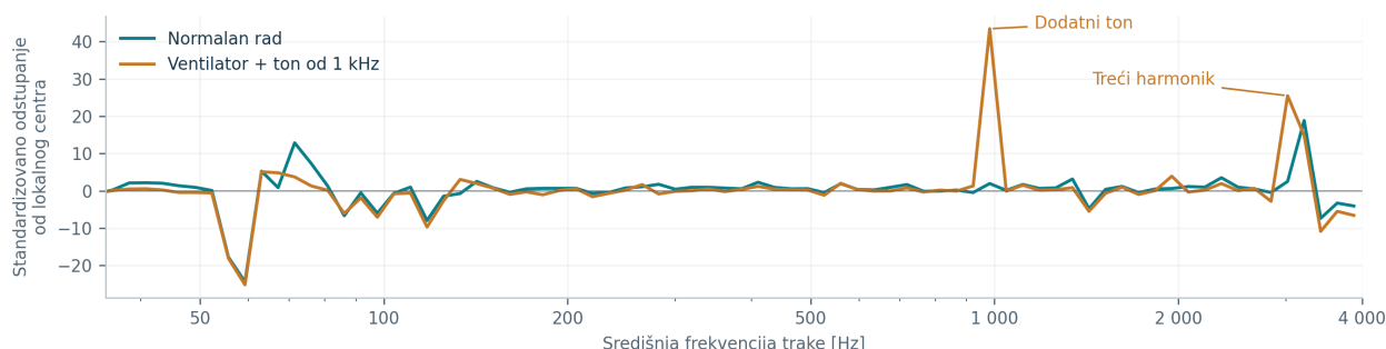
Slika 3. Odstupanje spektralnih karakteristika od lokalnog centra u fizičkoj probi. Pikovi oko 982 Hz i 3 021 Hz odgovaraju dodatnom tonu i trećem harmoniku. Prikazane su medijane po traci, a ne konačna ocjena alarma.
